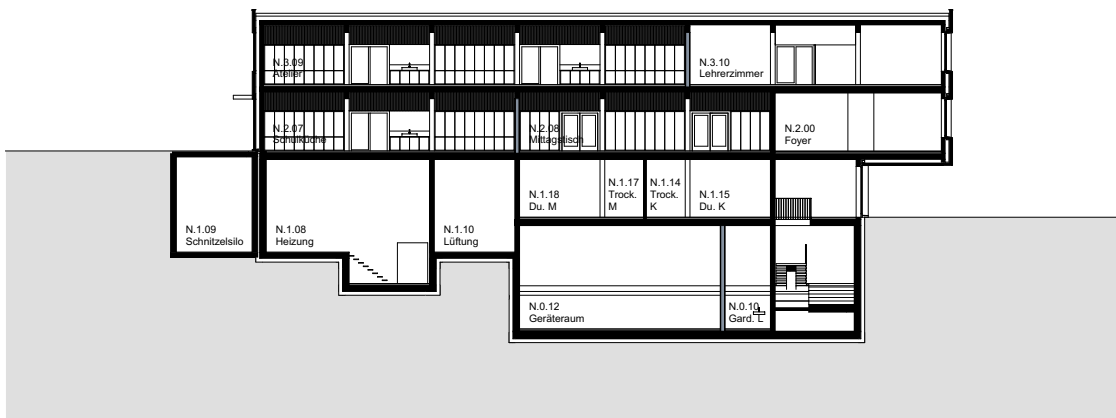
Schnitt N6
