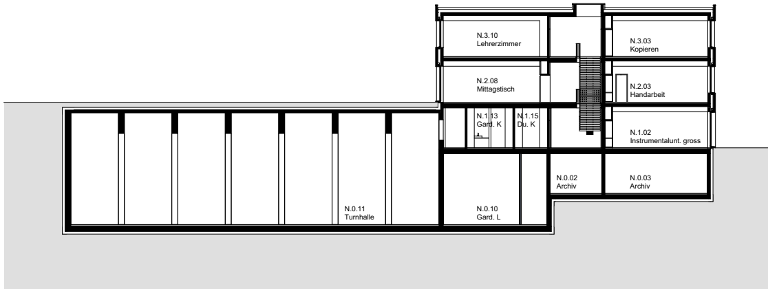
Schnitt N3
